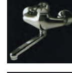
Art. 533 MISCELATORE MONOCOMANDO LAVELLO A PARETE Bocca di erogazione girevole mm. 200 o 300, eccentrici da 1/2" regolabili per interasse da mm.150 ± 15 WALL MOUNTED SINGLE LEVER SINK MIXER Swivel spout mm. 200 or 300, s-tailpieces with 1/2" connections, centre distance mm 150 ± 15
