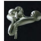
Art. 505 MISCELATORE MONOCOMANDO VASCA ESTERNO Deviatore automatico, duplex con flessibile mm.1500, eccentrici da 1/2" regolabili per interasse da mm. 150 ± 15 EXTERNAL SINGLE LEVER BATH MIXER Automatic diverter, duplex with shower hose mm. 1500, s-tailpieces with 1/2" connections, centre distance mm. 150 ± 15
